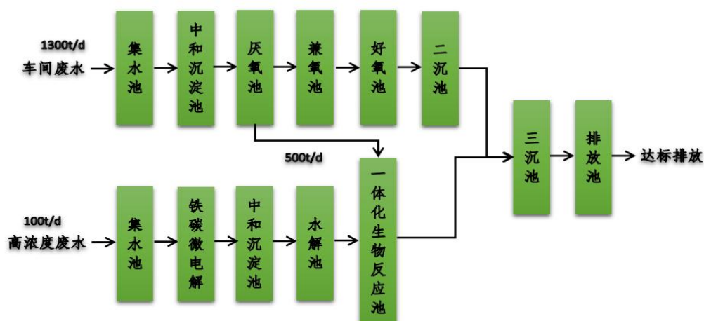
图 3.4-1 废水处理工艺流程图
