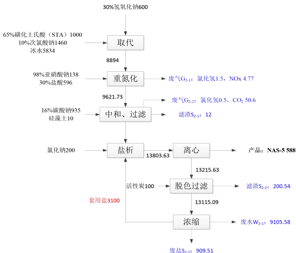
图 3.6-2 NAS-5 工艺流程图
