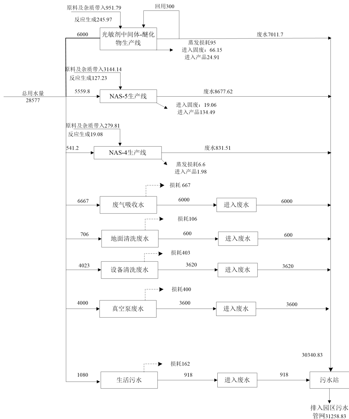
图 3.5-1 厂区水平衡图 单位: t/d
