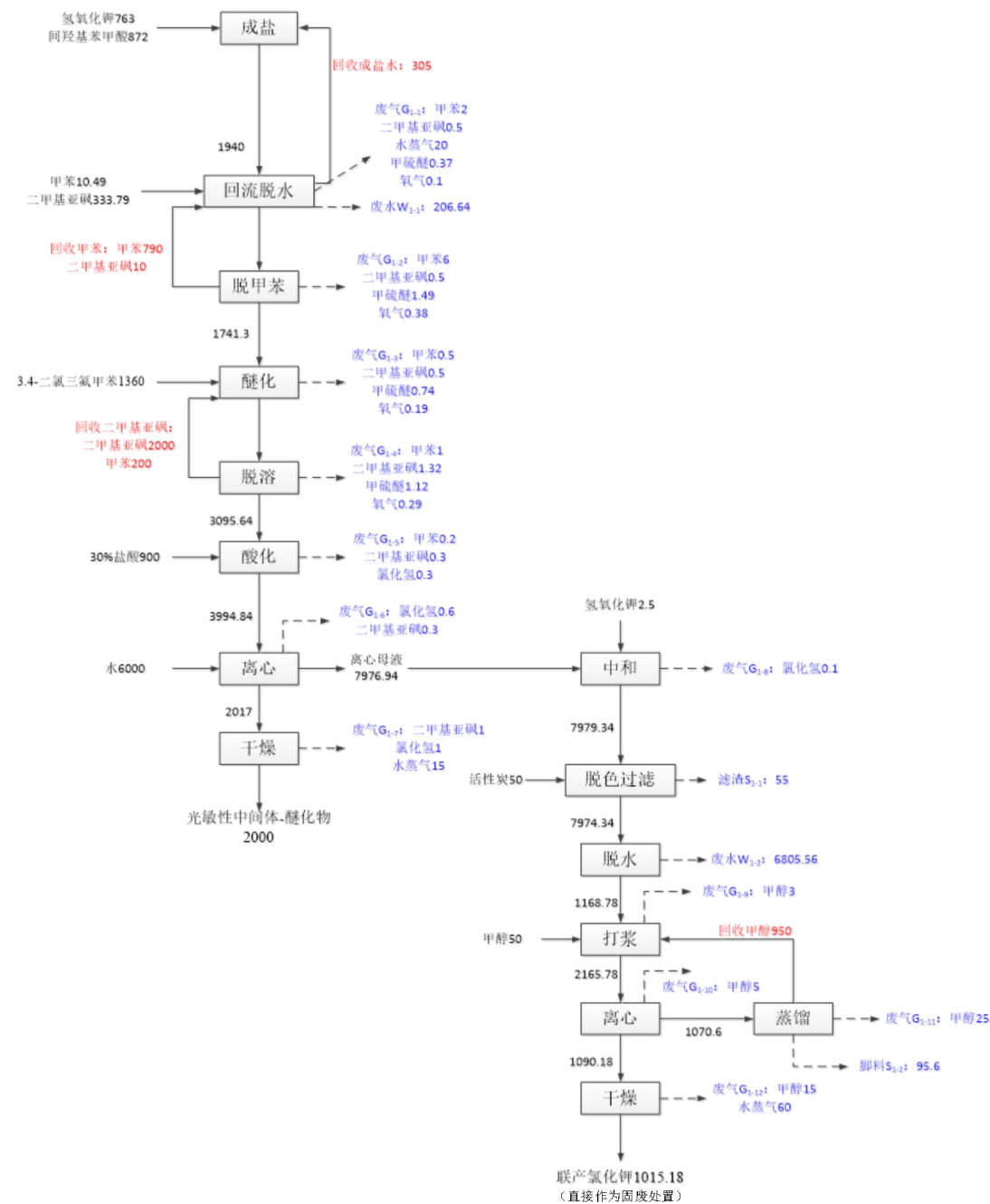
图 3.6-1 光敏性中间体-醚化物工艺流程图
