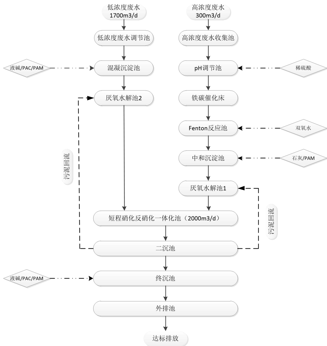
图 4.1-1 废水处理工艺流程图
