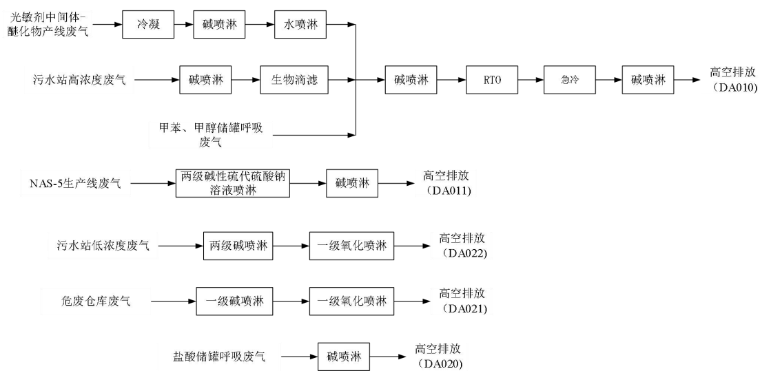
图 4.1-2 废气处理工艺流程图
